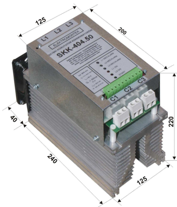
Rys. 1. Widok modułu SKK-404.50
