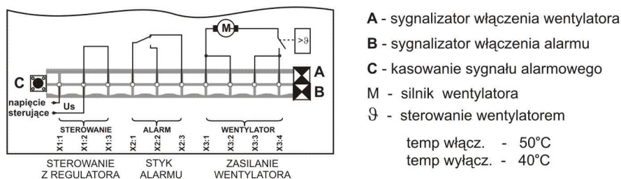
Rys. 2 Widok listwy obwodów sterowania SKK-404.50
