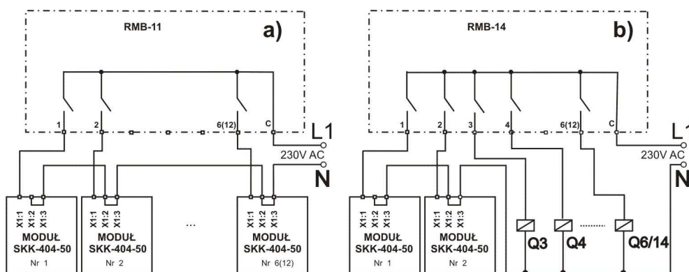
Rys. 3. Schemat sterowania modułów SKK-404.50
