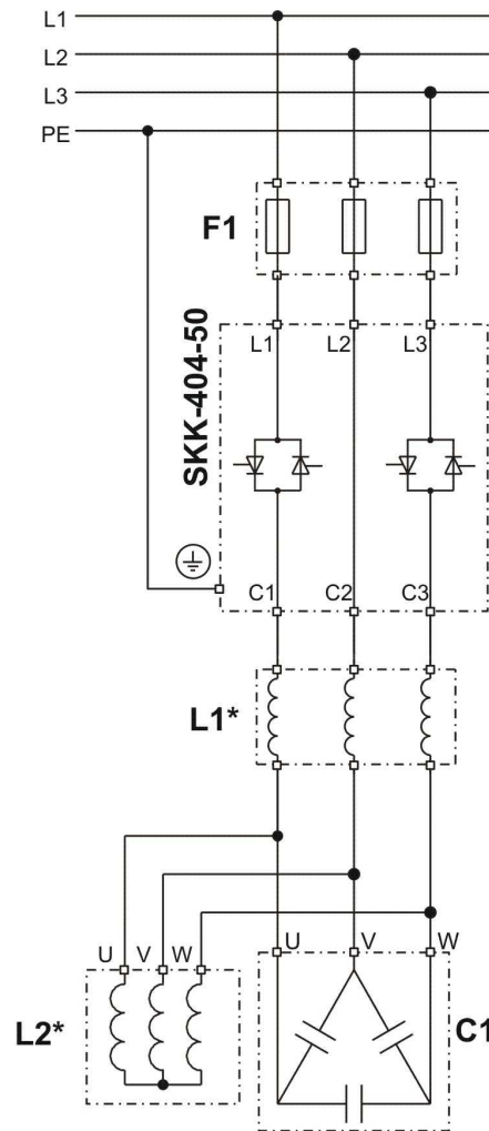
Rys. 4. Schemat ideowy członu baterii kondensatorowej z SKK-404.50
