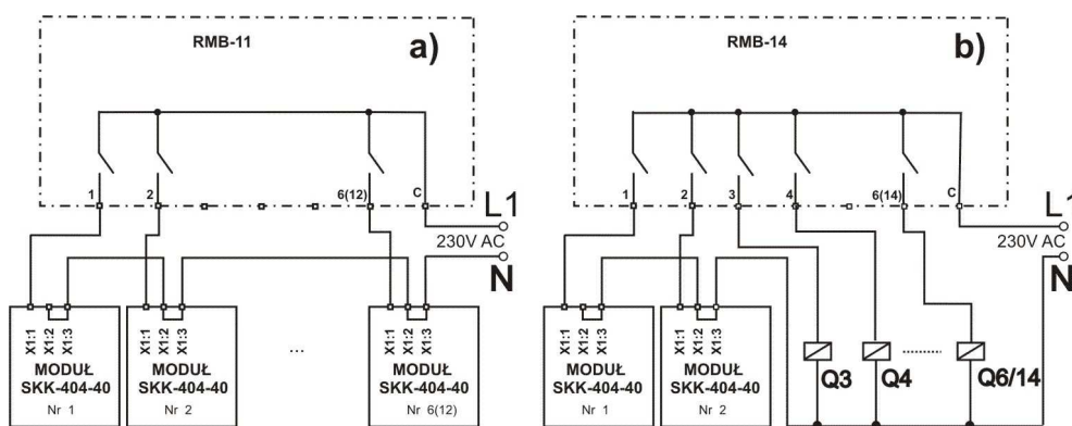
Rys. 3. Schemat sterowania modułów SKK-404.40
