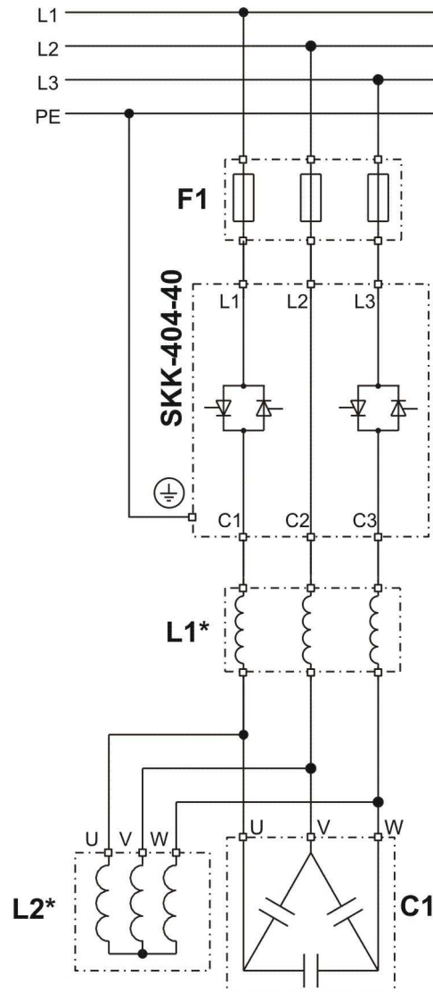
Rys. 4. Schemat ideowy członu baterii kondensatorowej z SKK-404.40
