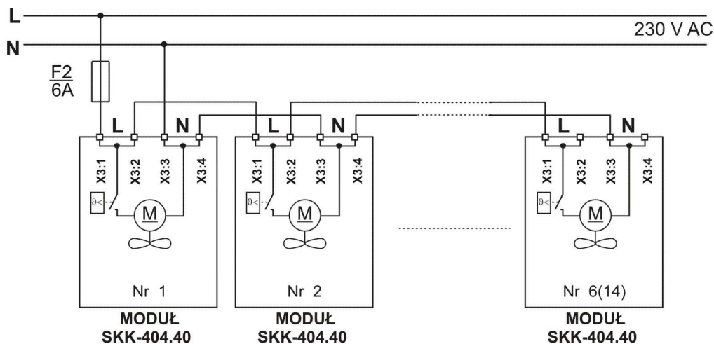
Rys. 5 Schemat podłączenia zasilania wewnętrznych wentylatorów.
