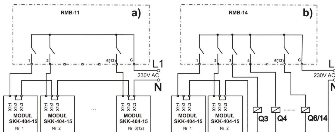
Rys 3. Schemat sterowania modułów SKK-404.15
