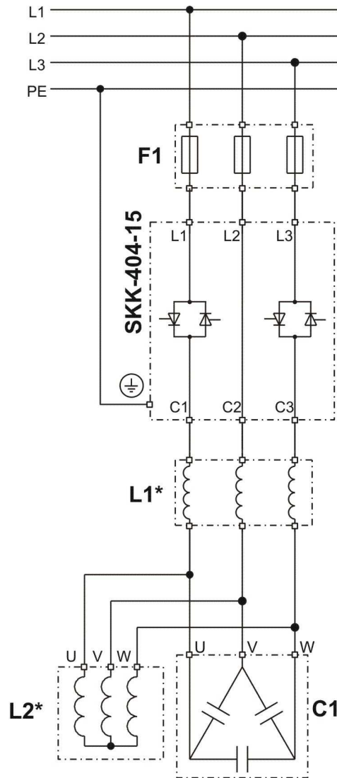
Rys. 4. Schemat ideowy członu baterii kondensatorowej z SKK-404.15 F1 - super szybkie bezpieczniki 50A L1* - obowiązkowa indukcyjność min. 20uH/50A L2* - reaktor rozładowczy kondensatora typu RRK-2, obowiązkowy ( R \leq 7,5k\Omega )
