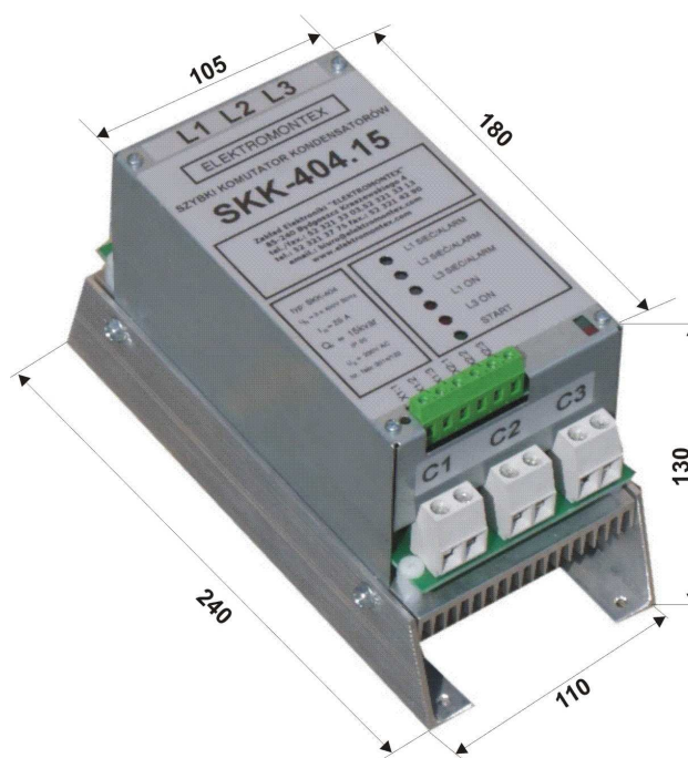
Rys. 1. Widok modułu SKK-404.15
