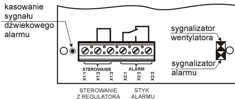
Rys. 2 Widok listwy obwodów sterowania SKK-404.15
